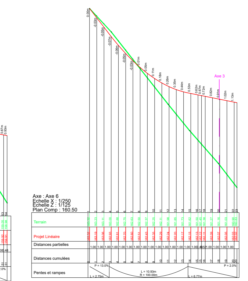
Axe 6 (1/250) :
