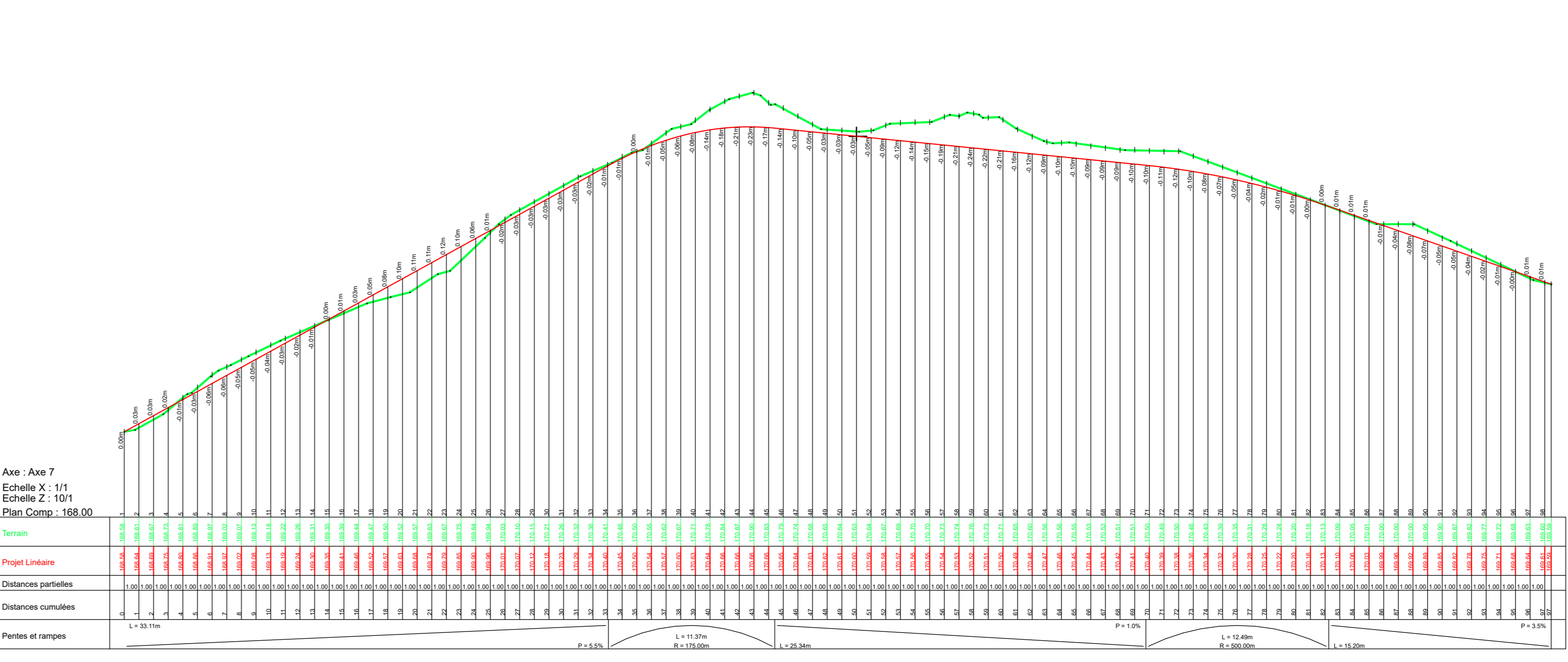
Axe 7 (1/250) :
