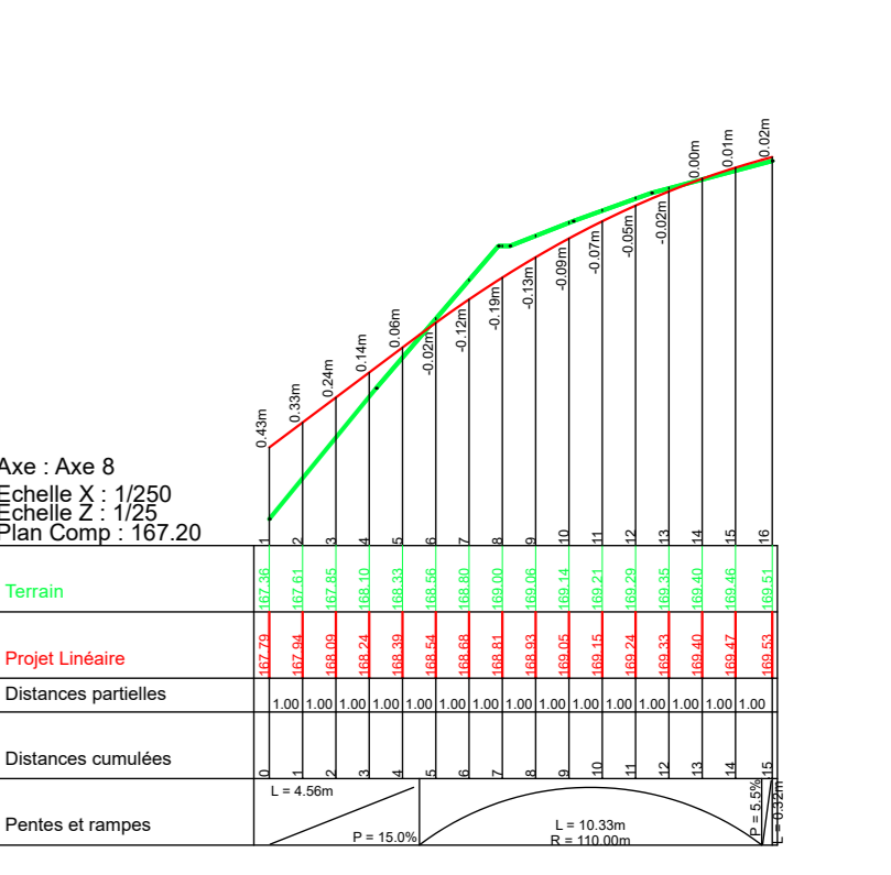
Axe 8 (1/250) :
