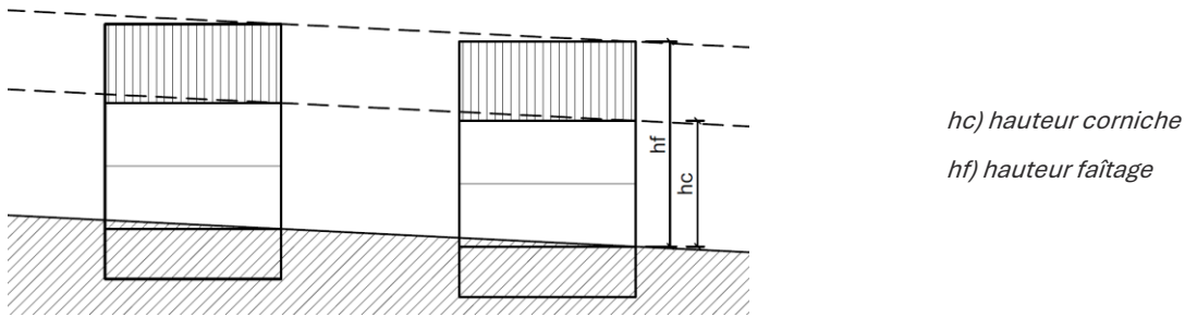
Figure 8 : Hauteurs des constructions dans le cas de la voirie desservante en pente
