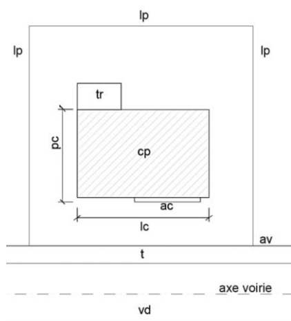
Figure 33 : Profondeur de construction
