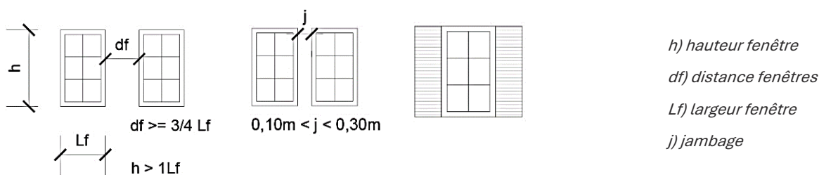
Figure 15 : Distance entre les ouvertures et volets rabattants
