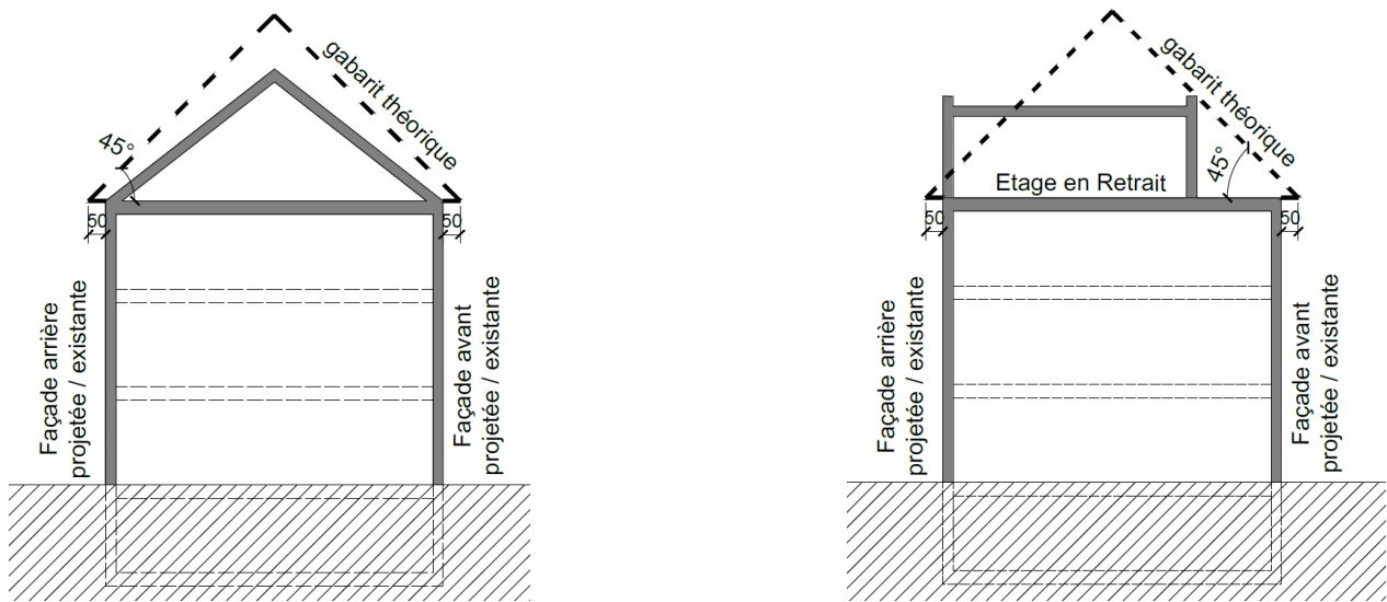
Figure 21 : définition du gabarit théorique pour toitures à deux versants et étages en retrait
