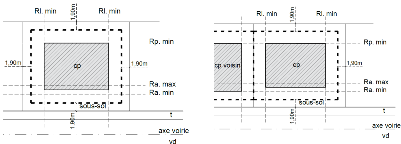
Figure 3 : Recul pour constructions en sous-sol en zones HAB-2 et MIX
