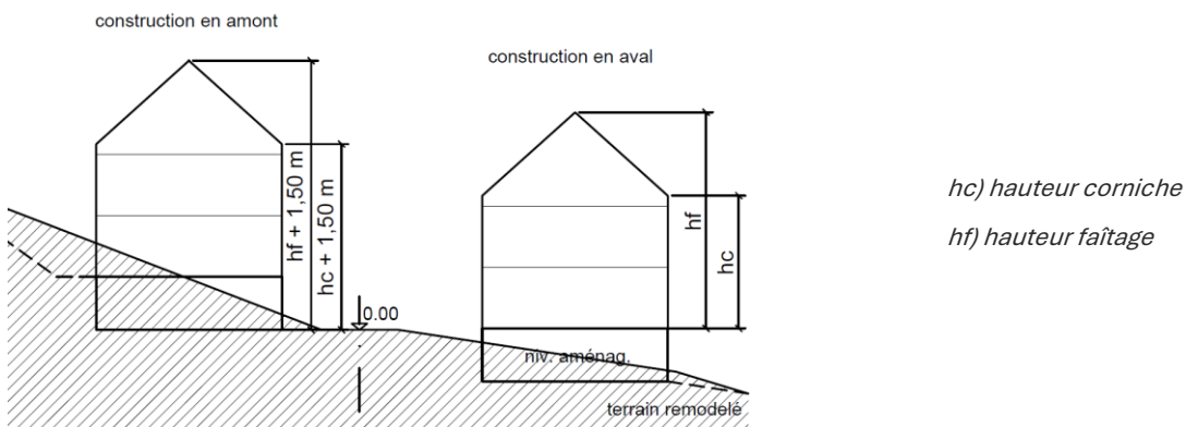
Figure 9 : Hauteurs des constructions dans le cas du terrain en pente
