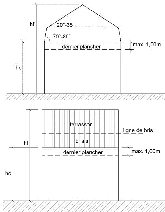
Figure 4 : Toiture mansardée
