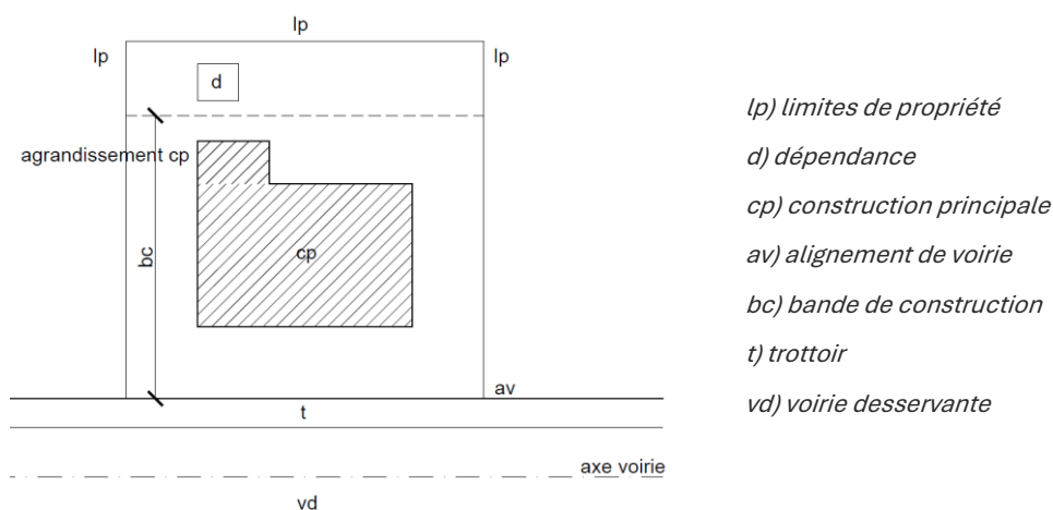
Figure 20 : Bande de construction
