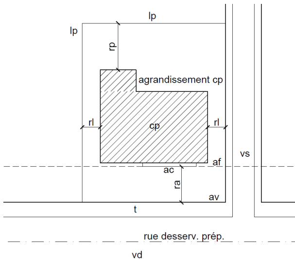
Figure 32 : Reculs pour propriétés sises aux angles de rues
