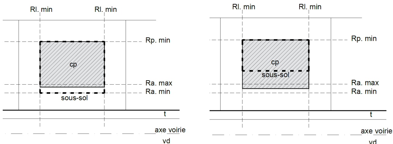
Figure 2 : Recul pour constructions en sous-sol en zone HAB-1
