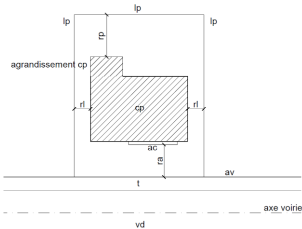
Figure 29 : Marges de reculement
