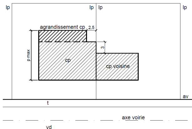
Figure 1 : Construction accolée à une construction existante
