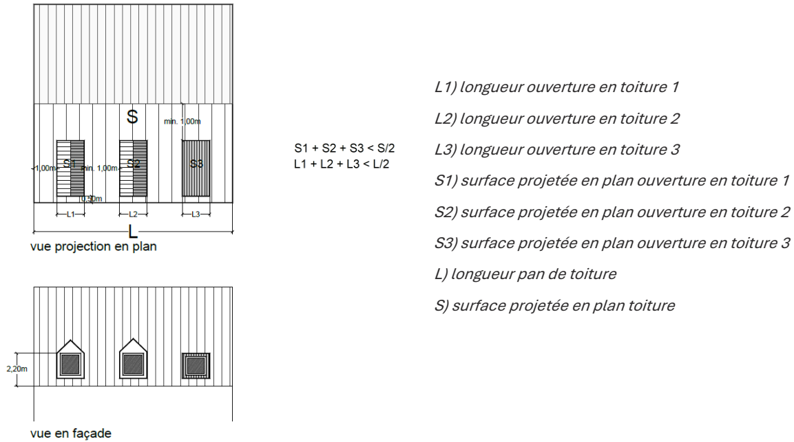
Figure 5 : Ouvertures en toiture
