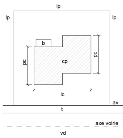
Figure 34 : Profondeur de construction pour façades opposées non-parallèles
