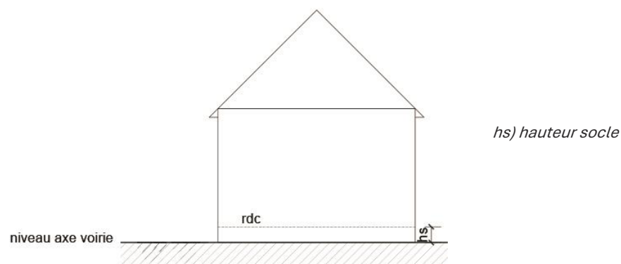
Figure 28 : Hauteur du socle
