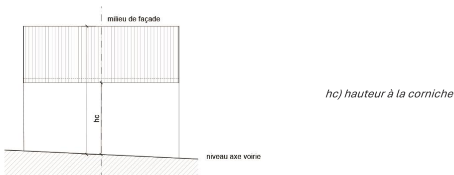
Figure 24 : Hauteur à la corniche dans le cas de voirie en pente
