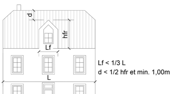
Figure 14 : Frontons sur les façades du Noyau de Mertert
